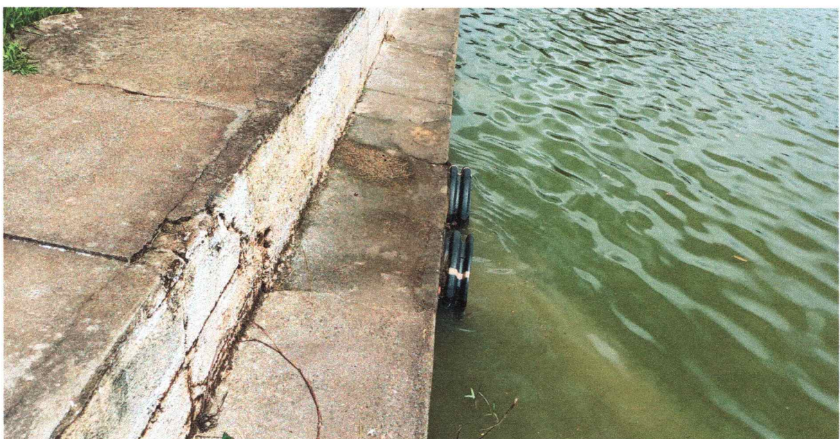
Figura 04 -. Vista do local ilustrando tubos para permitir a vazão da água do local, quando apresenta aumento em seu armazenamento.
